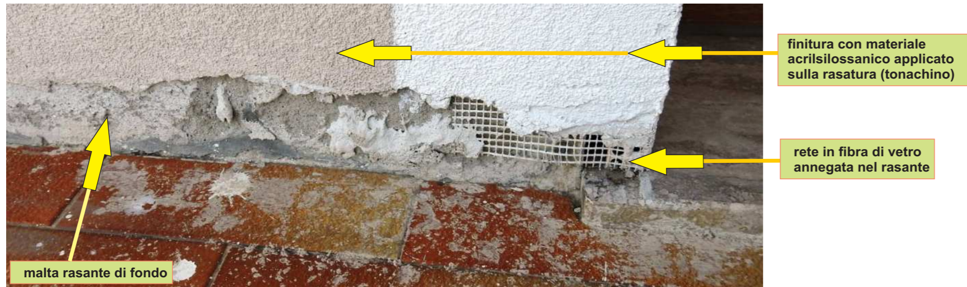
Foto N°32 - Particolare esecutivo della rasatura e finitura delle pareti esterne: si può notare la rete rinforzante in fibra di vetro annegata nel rasante ed il soprastante strato di finitura con tonachino premiscelato del tipo acrisilossanico
