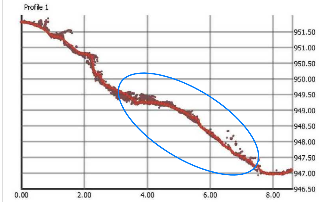
Fig. 2 - Profilo longitudinale della scarpata di cui alla Figura 2 (in ascisse sono indicate le lunghezze, in ordinate le altezze)
